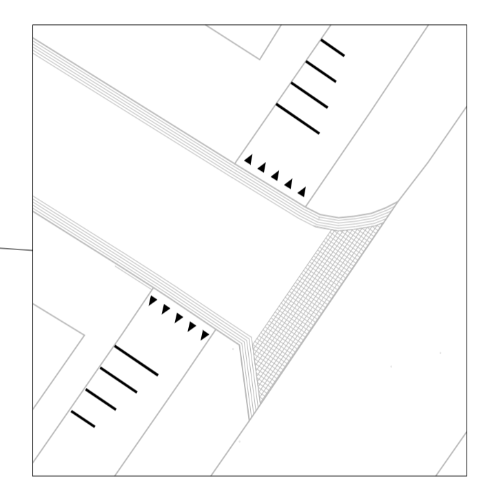
UDSNIT 1:200
