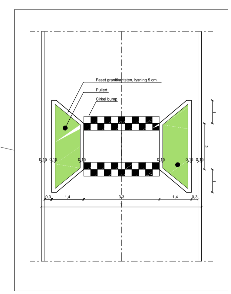
UDSNIT 1:100
